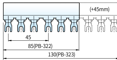
MMS-32S+PB-32 PB-322 (2단자용), PB-323 (3단자용) PB-324 (4단자용), PB-325 (5단자용)
