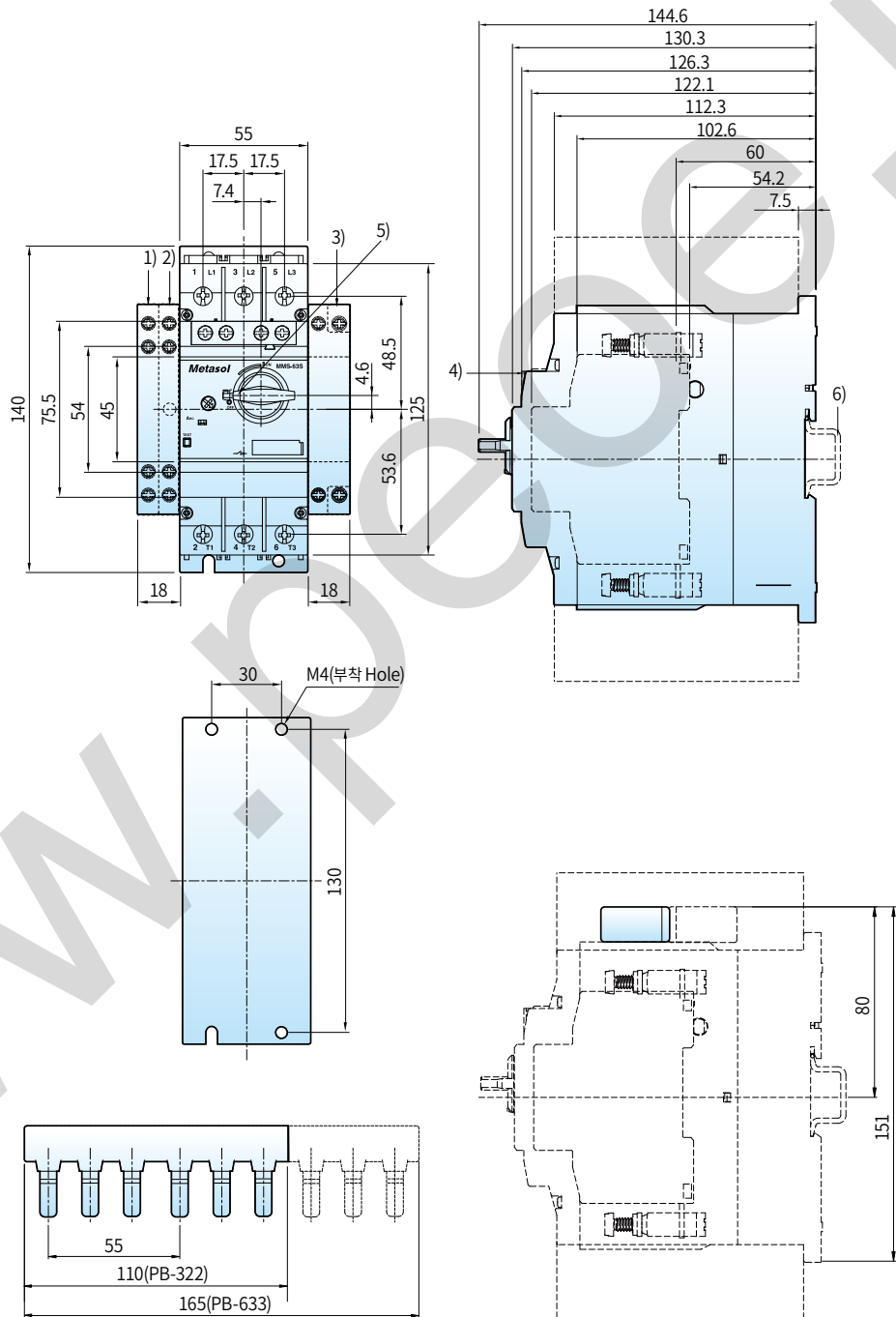
MMS-63S/H/Hi+PB-63 PB-632 (2단자용), PB-633 (3단자용)
