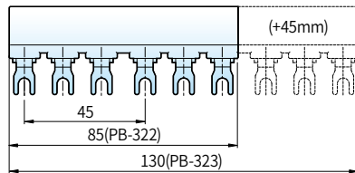
MMS-32H/HI+PB-32 PB-322 (2단자용), PB-323 (3단자용) PB-324 (4단자용), PB-325 (5단자용)
